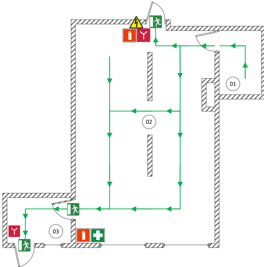
Експлікація приміщень
